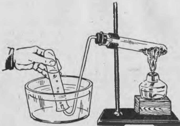
103 сур. Кислород чыгъарыгъа прибор.
