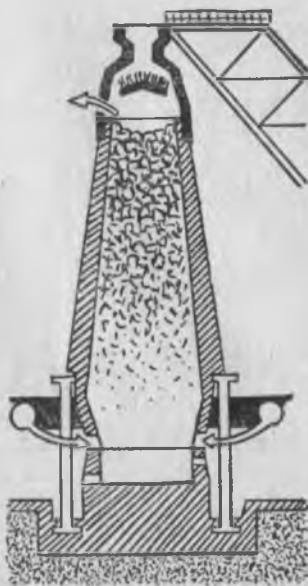
53 сур. Домна печь (разрезинде):
