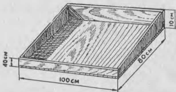
184 сур. Кумдан модель этерге джюрюютюлген агъач ящик.
