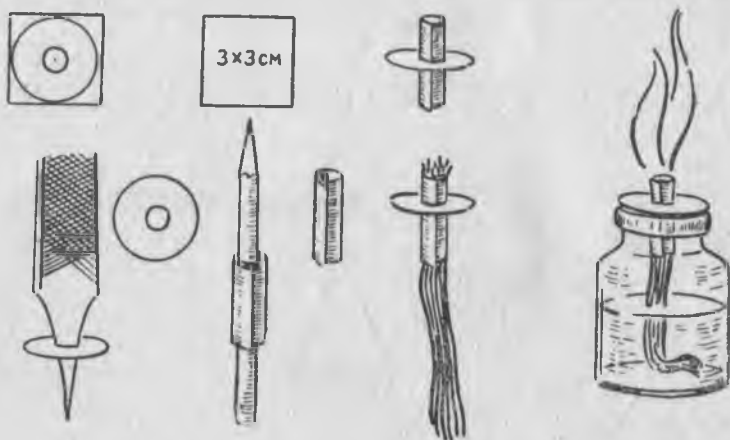
183 сур. Спирт лампачыкны кыалай этедиле.
