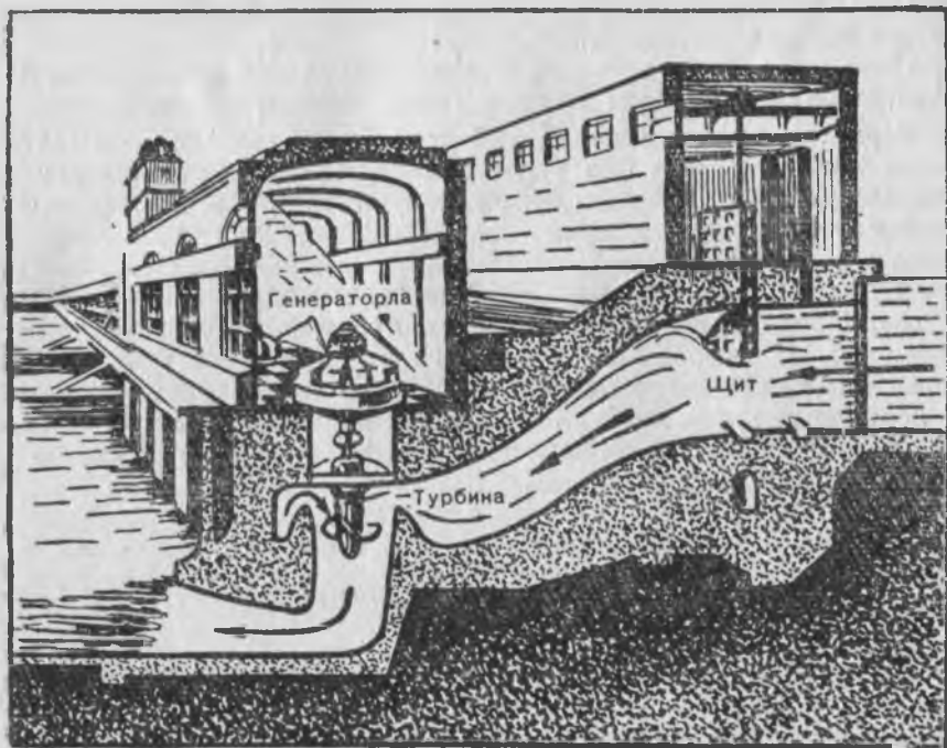
61 сур. Гидроэлектростанцияны разреза.
