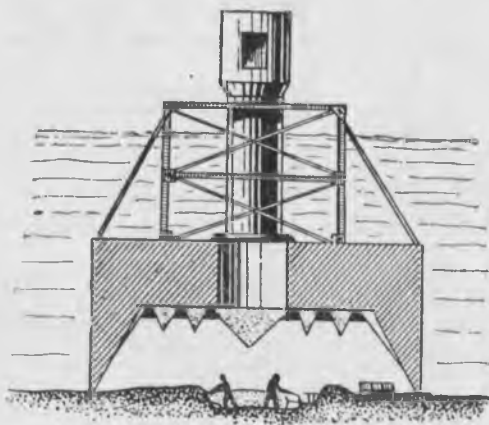
87 сур. Адамла сууну тюбюнде ишлейдиле.
